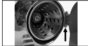
Bewegliche Abschirmung mit Mikroschalter
